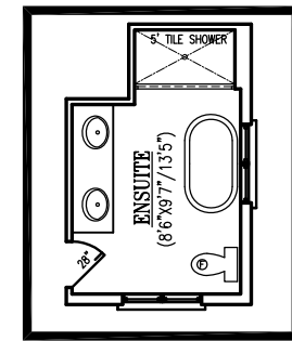
ENSUITE - OPTION 2
